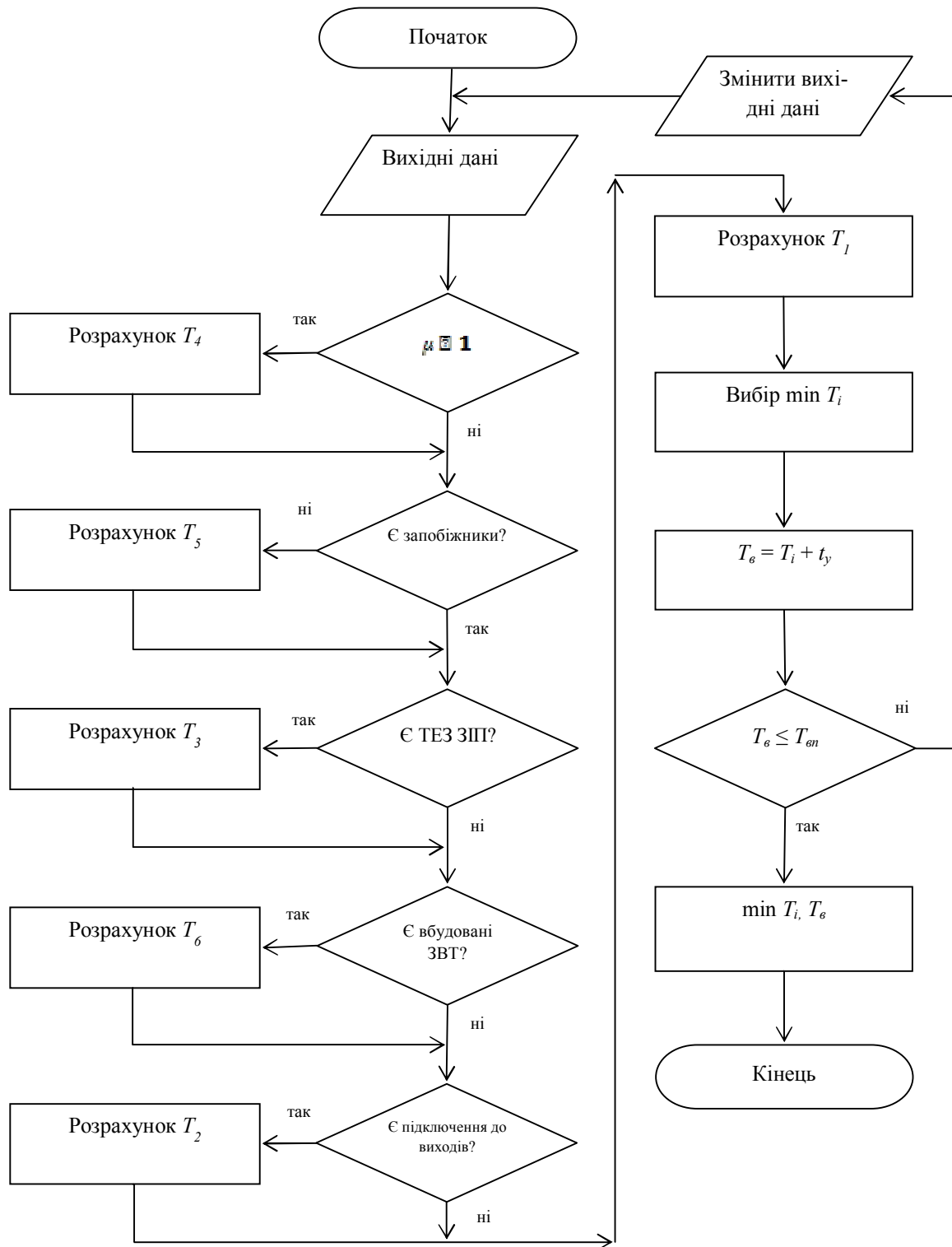
Рис. 3. Блок-схема алгоритму вибору варіанту діагностування
