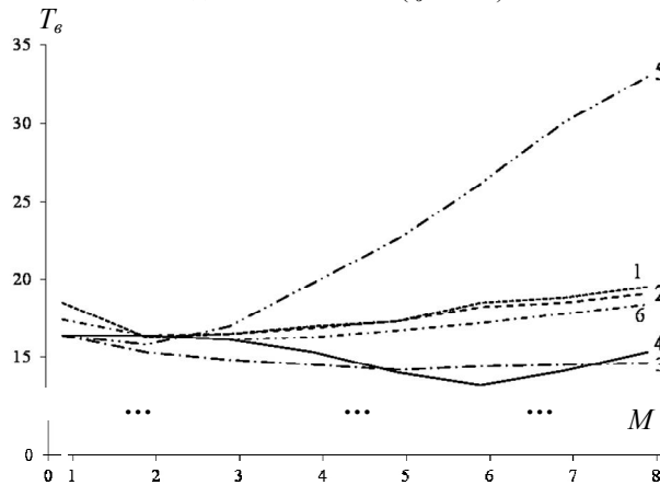
Рис. 2. Залежності середнього часу відновлення від кількості блоків ( t_6 = 2 \text{ хв} )
