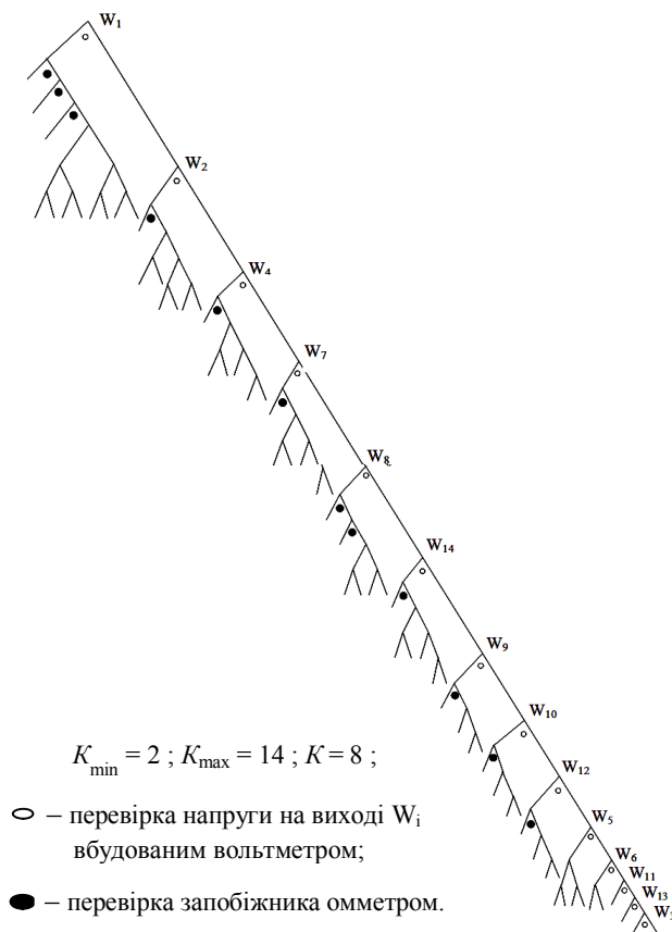
Рис. 4. Умовний алгоритм діагностування блоку електроживлення БЗ-28
