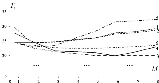
Рис. 1. Залежності середнього часу відновлення від кількості блоків ( t_6 = 3 \text{ хв} )
